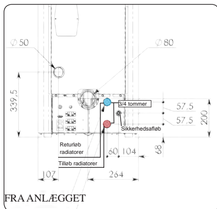
Fig. 12-A HR100 / HRV120
